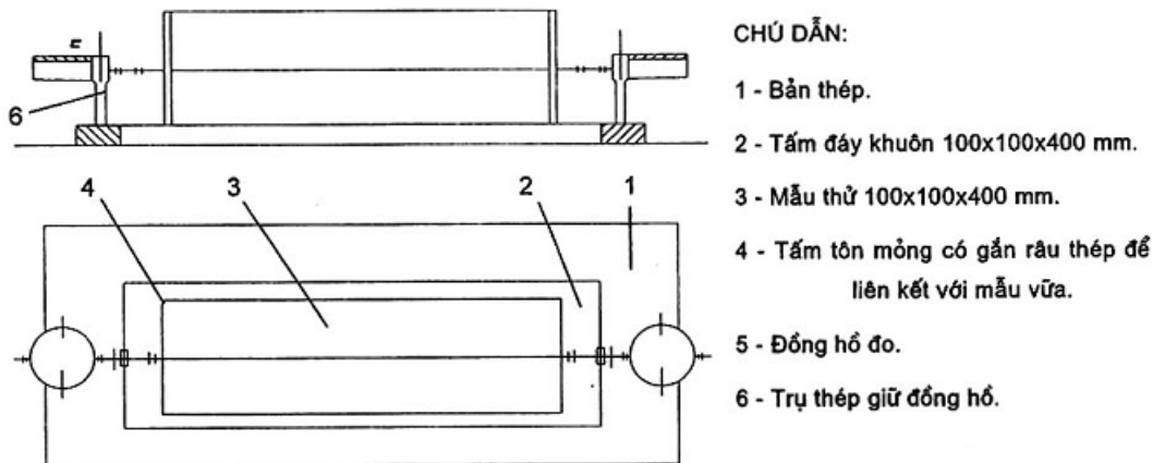
Hình 2 - Sơ đồ thí nghiệm xác định sự thay đổi chiều dài mẫu vữa đã cứng
